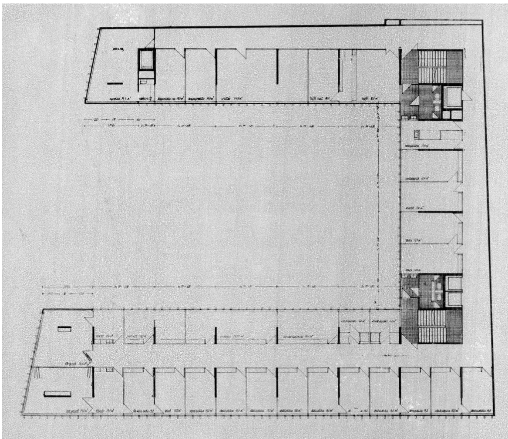
15.kép. Általános emeleti alaprajz. (első, sűrű ablakosztásos változat).
